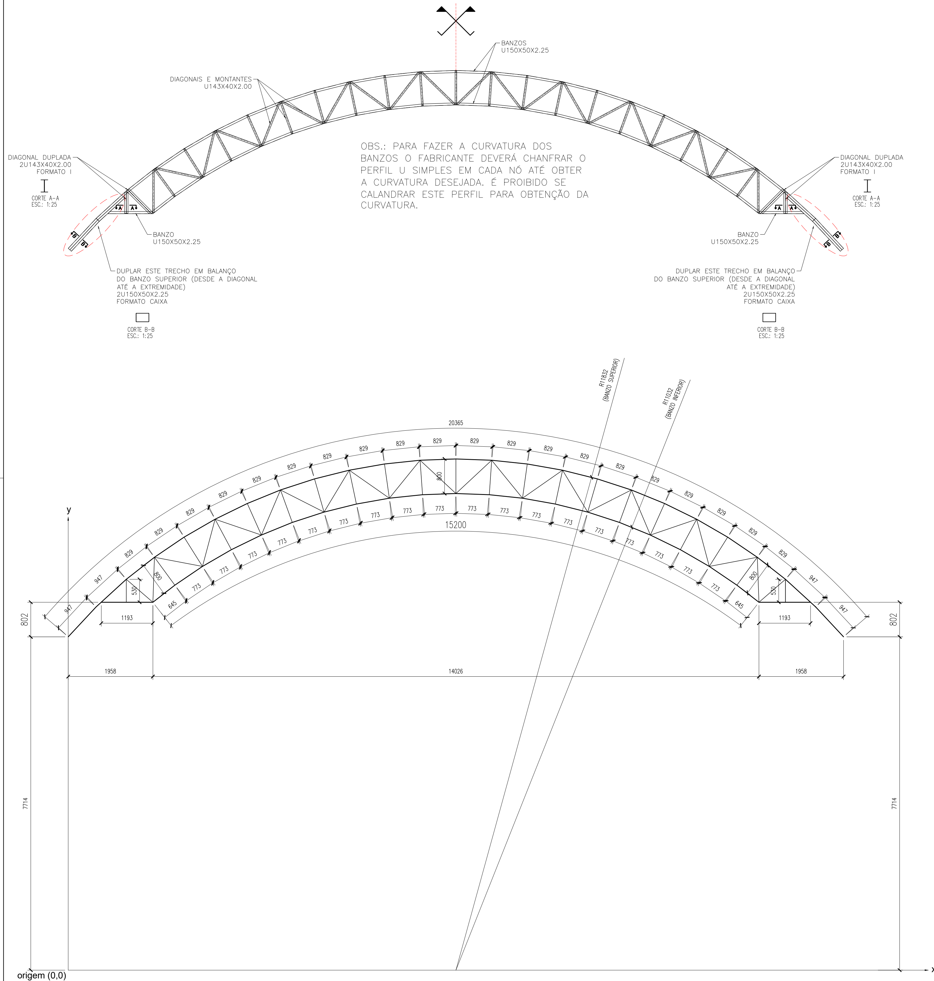
FABRICAÇÃO DA TRELIÇA TR01 (x5) ESC.: 1:50
