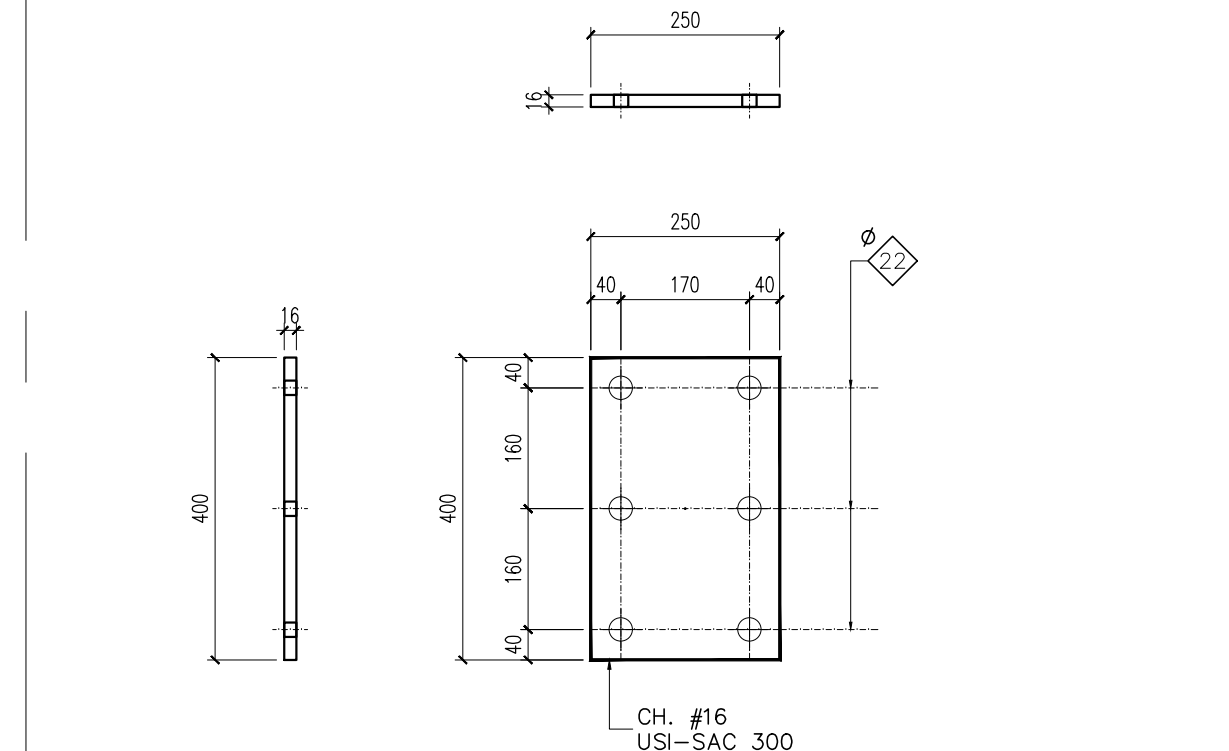
CH.BASE (x10) - LAMINADO 400x250 #16 ESC.: 1:10
