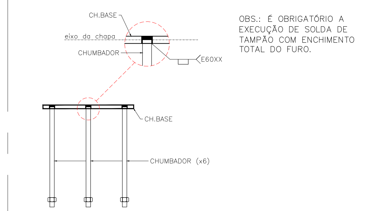
FABRICAÇÃO DOS INSERTS METÁLICOS (x10) SEM ESC.
